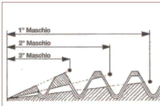
Maschi a mano in serie di tre pezzi
